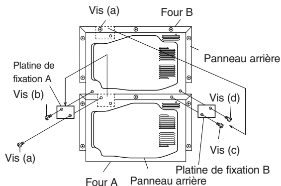
Figure A: Installation de deux fours
