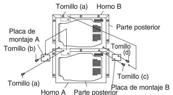
Figura A. Cómo instalar dos hornos
