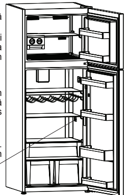
Lämpötilasensorin alue
