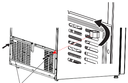
Plastmasa attāluma regulēšanai starp sienu un ledusskapi
