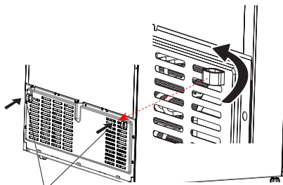
Пластмасов водач за регулиране на разстоянието между задната стена и хладилника
