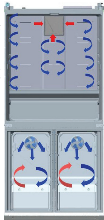
Сини стрелки: Издухване на студения въздух Червени стрелки: Връщане на топлия въздух
